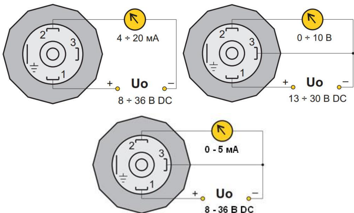
Малюнок 2 – Електрична схема підключення перетворювача
