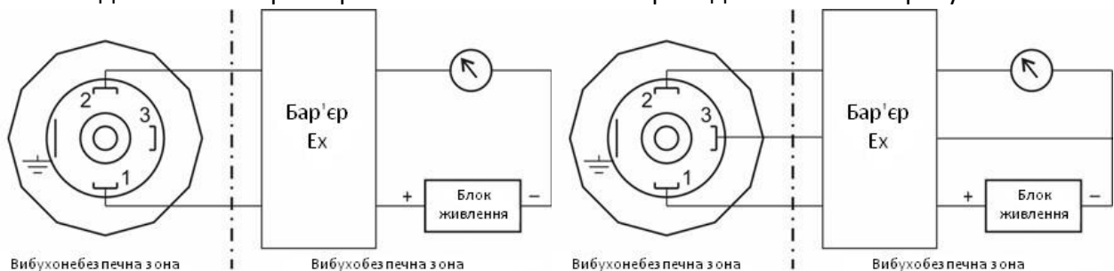
Малюнок 3 – Схеми електричних підключень перетворювачів в іскробезпечному виконанні
