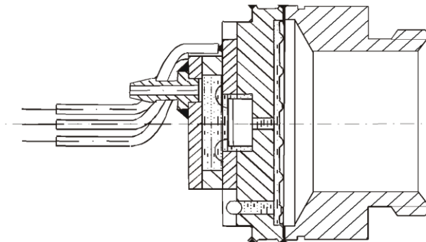
Малюнок 1 – Будова вимірювального модуля
