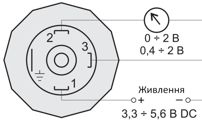
Малюнок 3 – Електрична схема підключення перетворювачів в іскробезпечному виконанні
