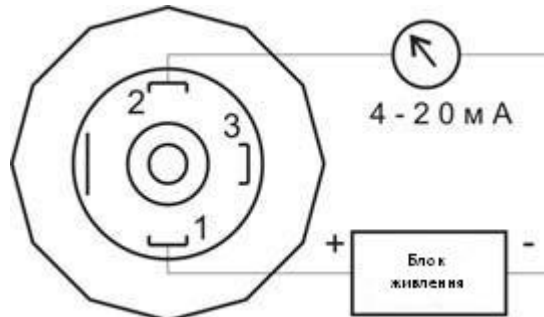
Малюнок 2 – Електрична схема підключення перетворювачів
