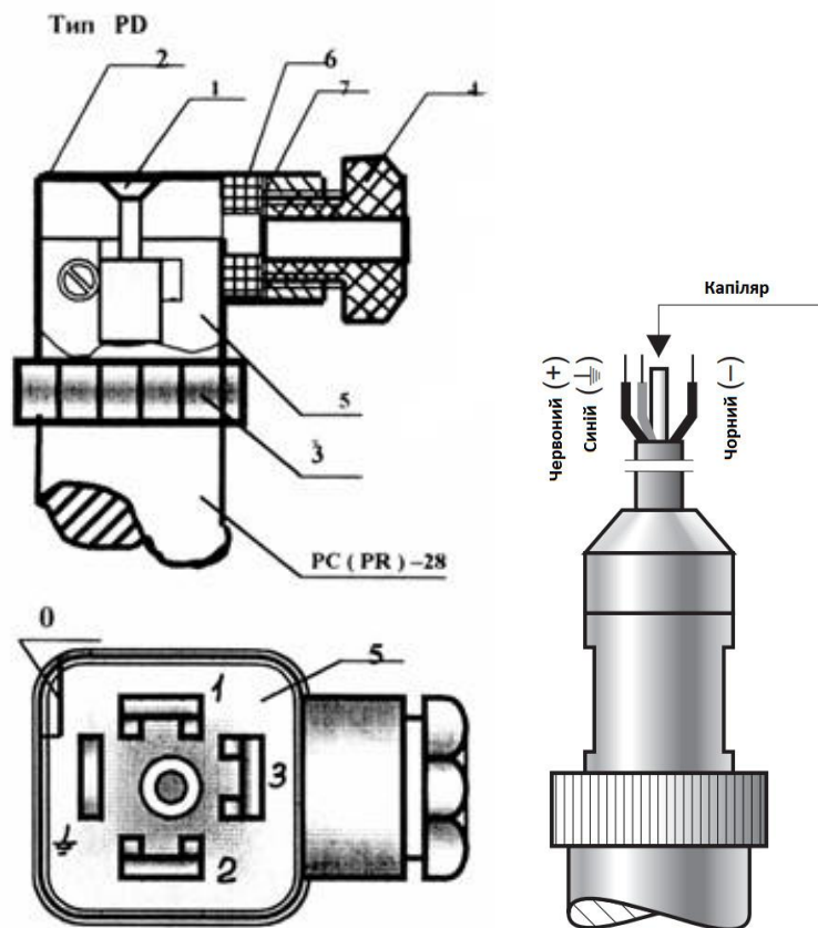
Малюнок 4 – Види електричних приєднань (PD, PK)
