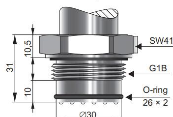
Тип CG1 Штуцер G1" із лицевою мембраною Діапазон від -10...10 кПа до 0...7 МПа Матеріал змочуваних частин: 316L
