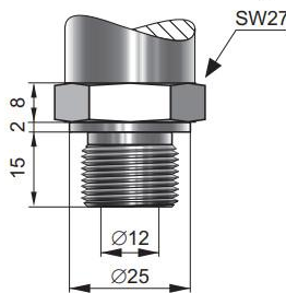
Тип P Штуцер M20x1,5, отвір Ø12 Тип GP Штуцер G1/2", отвір Ø12 Матеріал: 316L Hastelloy C-276 - спец викон.
