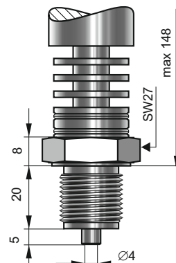
Тип RM Радиатор со штуцером М
