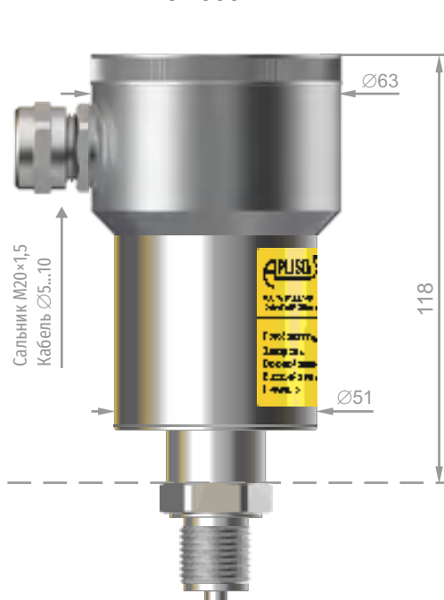
Пример со штуцером типа М
