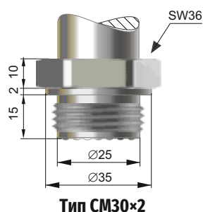
Тип CM30×2 Штуцер M30×2 с лицевой мембраной Диапазоны от -10...10 кПа до 0...7 МПа Материал смачиваемых частей: 316L стандарт; Hastelloy C-276 – спец исп.
