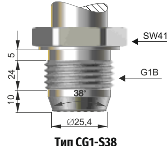
Тип CG1-S38 Штуцер G1" конус 38 гр. с лицевой мембраной диап. 0...100 кПа Материал смачиваемых частей: 316L, Hastelloy C-276 – спец исп.
