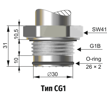
Тип CG1 Штуцер G1" с лицевой мембраной Диапазоны от -10...10 кПа до 0...7 МПа Материал смачиваемых частей: 316L стандарт; Hastelloy C-276 – спец исп.
