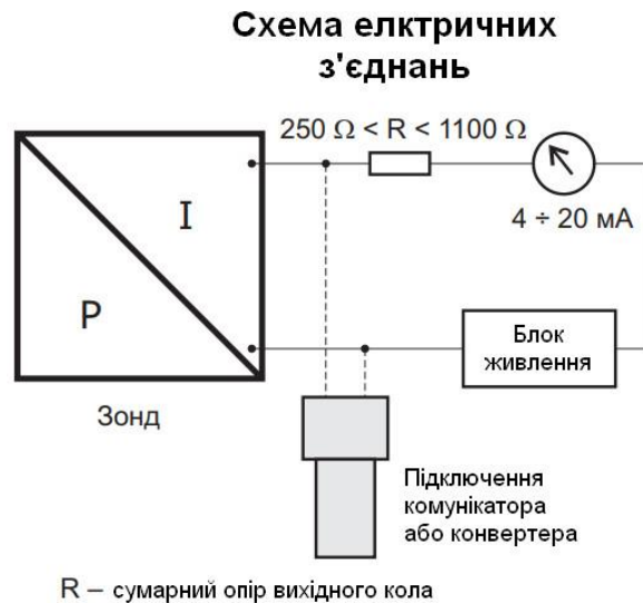
Малюнок 2 – Схема електрична підключення перетворювача
