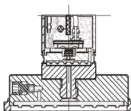
Малюнок 1 – Будова вимірювального модуля
