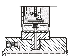
Малюнок 1 – Будова вимірювального модуля
