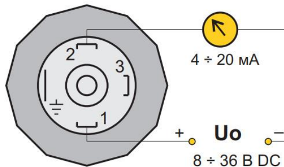
Малюнок 2 – Електрична схема підключення перетворювача
