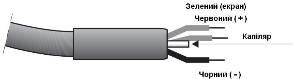
Малюнок 3 – Електричне приєднання
