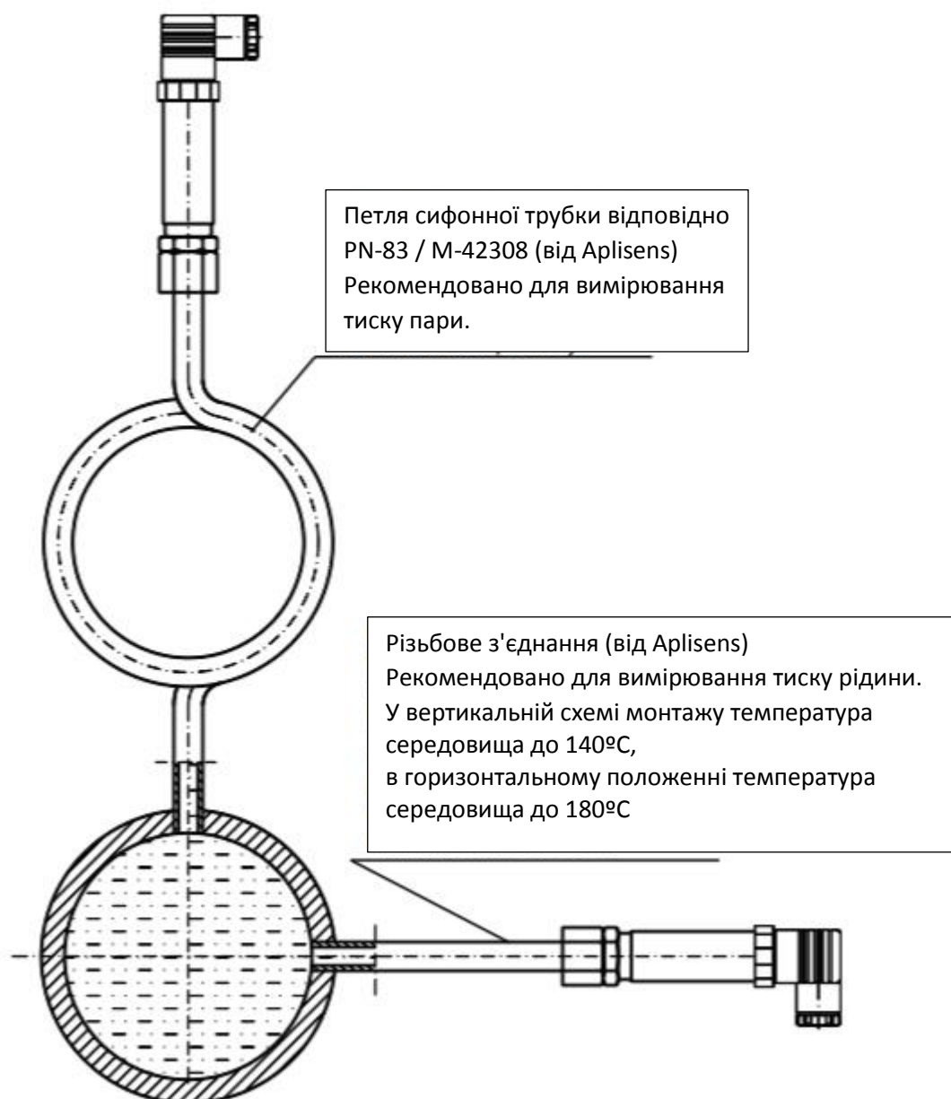
Рис.15. Приклад поділу перетворювача від впливу високої температури
