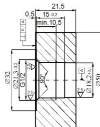
Рис.12г. Кільце для роботи зі з'єднанням типу CG1 / 2 з мембраною Матеріал - сталь 1.4404 (316L) Код замовлення: Роз'єм CG1 / 2
