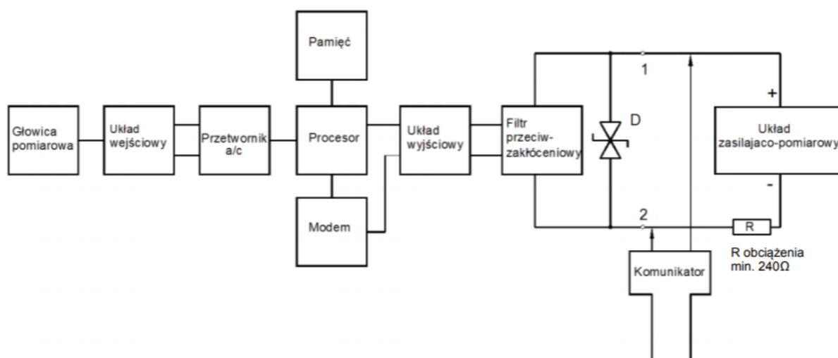
Рис.1. Структурна схема перетворювачів серії PC-28.SMART
