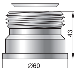
Соединитель Level с прокладкой
